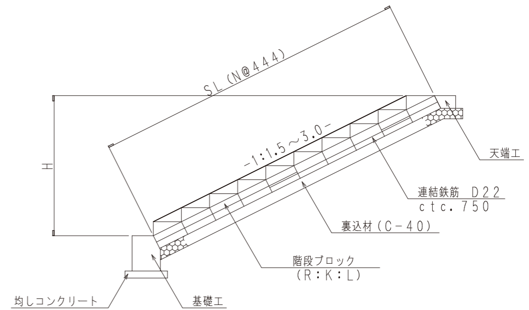
勾配 1割5分～3割 通常タイプ
