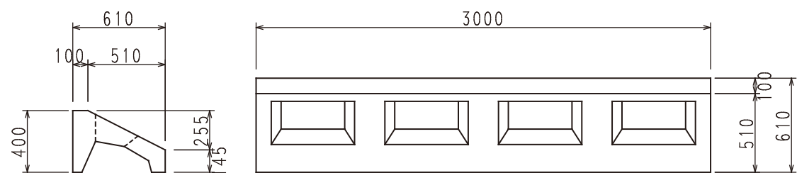
ブロック控長55cm用(5分)
