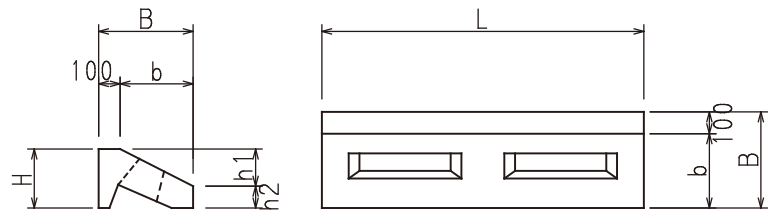
ブロック控長35cm用
