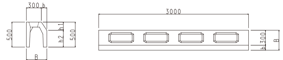
張ブロック控長20cm用
