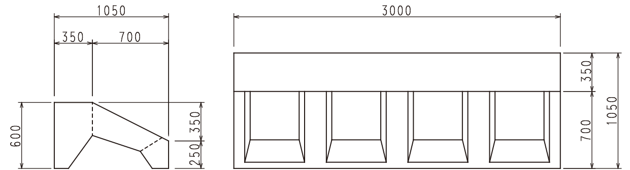
ブロック控長75cm用(5分)
