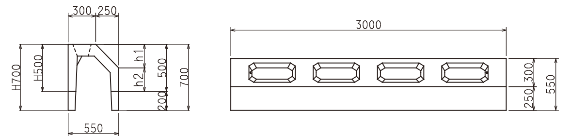
張ブロック控長35cm用
